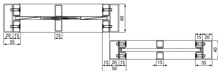
1-skrzydłowe stalowe drzwi loftowe z naświetlem bocznym, przekrój poziomy
