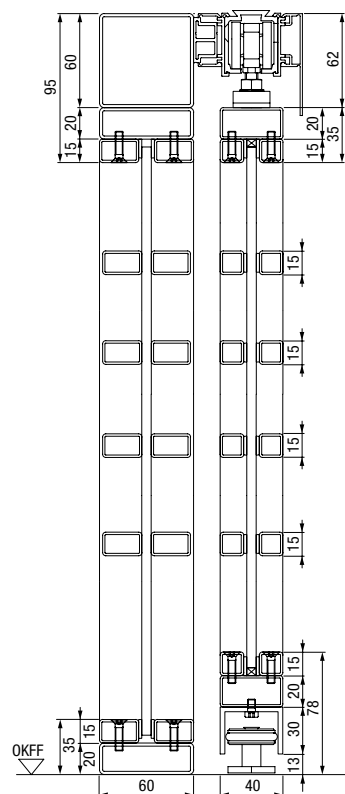
1-skrzydłowe stalowe drzwi loftowe z naświetlem bocznym, przekrój pionowy
